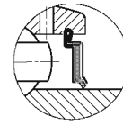
F密封 (+后缀F)
