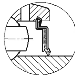
F密封 (+后瓣F)
