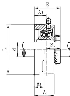
UKFL2+H 带紧定套
