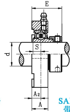
SBLFTC2G 带顶丝
