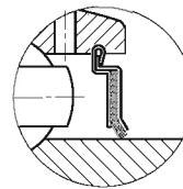
F密封 (+后缀F)
