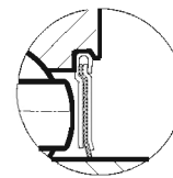
F密封 (+后缀F)
