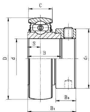
SA0 带偏心套外球面球轴承
