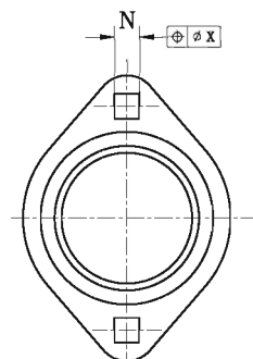
PFL
