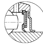
双层密封
