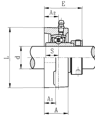
NAFL3 带偏心套
