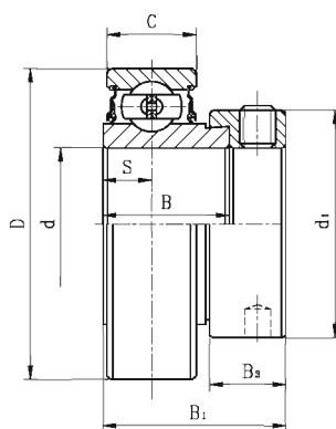
CSA1 CSA2 带偏心套外圆柱面球轴承
