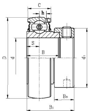
GRA2 带偏心套外球面球轴承
