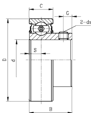
CSB2 带顶丝外圆柱面球轴承
