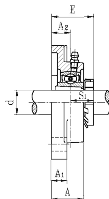
UKF3+H 带紧定套
