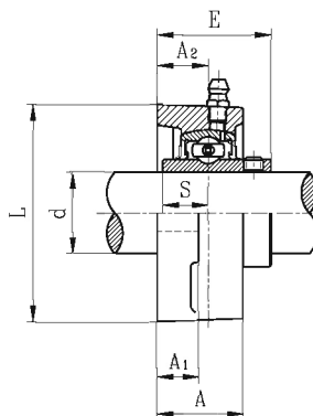
UCFL3 带顶丝
