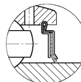
F密封 (+后辮F)
