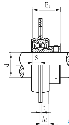
SBPFT2 带顶丝
