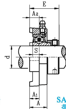
SBPFTD2G 带顶丝
