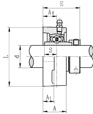
NAFLU2 带偏心套
