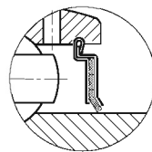
F密封 (+后缀F)
