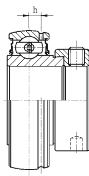
SA2G 再润滑型
