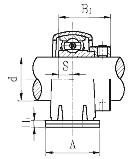
SAPP2 带偏心套
