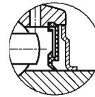
双层密封
