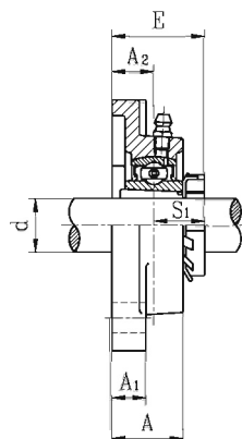
UKF2+H 带紧定套
