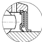
双层密封
