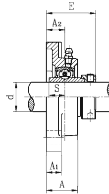
NAF3 带偏心套
