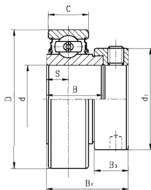
RA2 带偏心套外圆柱面球轴承
