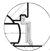
UC2T 带锁紧套外球面球轴承
