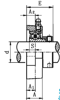
SBLF2G 带顶丝
