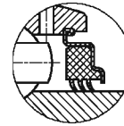
三层密封 (+后缀R3)
