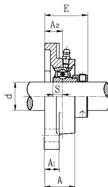
SAF2G 带偏心套
