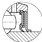
双层密封
