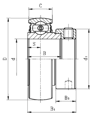
SA2 带偏心套外球面球轴承
