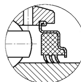
三层密封 (+后辮R3)
