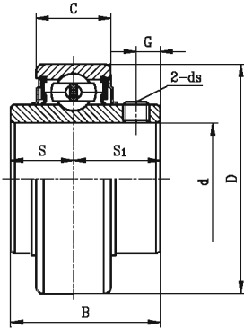
RB2
