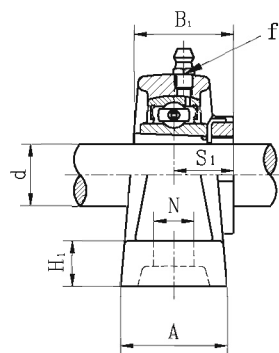
UKP200M+H 带紧定套
