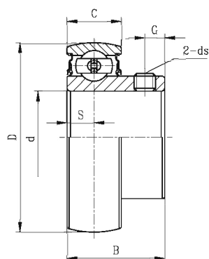
SB2 带顶丝外球面球轴承
