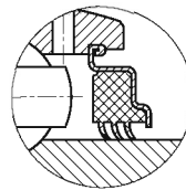
三层密封 (+后缀R3)
