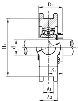
UKT3+H 带紧定套
