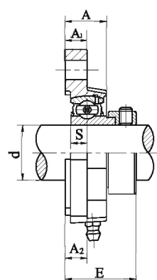
SAFCT2G 带偏心套
