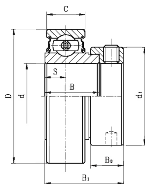
CSA0 带偏心套外圆柱面球轴承
