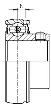
SB2G 再润滑型
