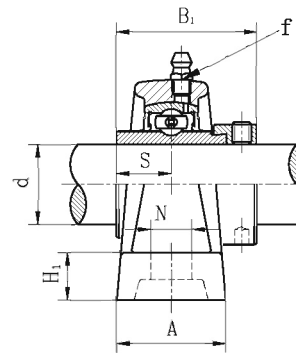
NAP200M 带偏心套
