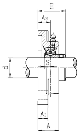
SBF2G 带顶丝
