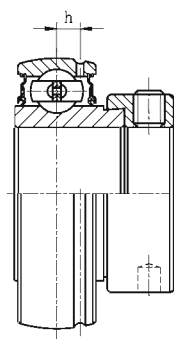
GRA2G 有油槽型
