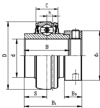
HC2
