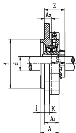
UKFC2+H 带紧定套
