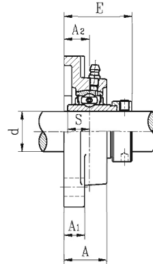
NAFU2 带偏心套
