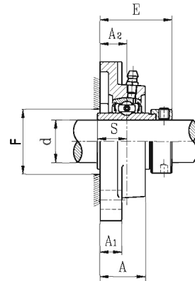
NAF2 带偏心套
