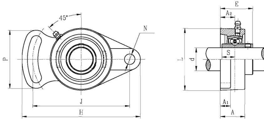
UCFA2 带顶丝
