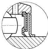
双层密封
