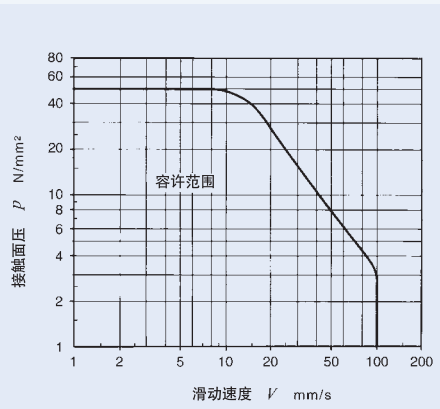
图4 不加油式杆端关节轴承杆端的 pV 曲线图
