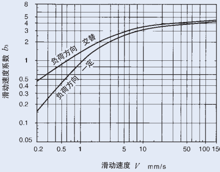
图3 加油式杆端关节轴承的滑动速度系数
