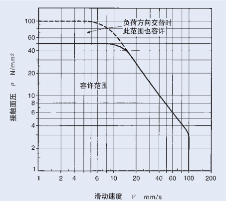
图4 不加油式关节轴承的pV曲线图
