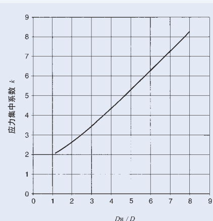
图7 应力集中系数
