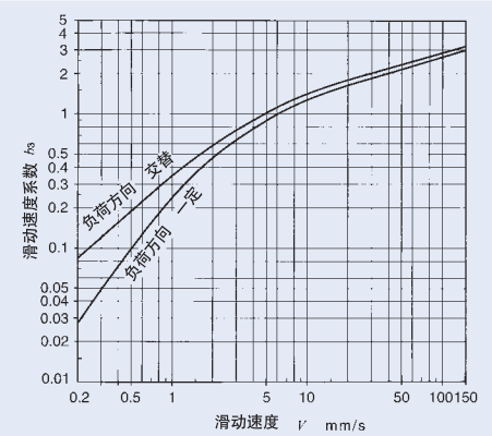
图3 滑动速度系数
