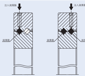
图6 加油方法
