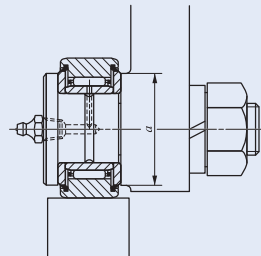
图1 安装部侧面的高度
