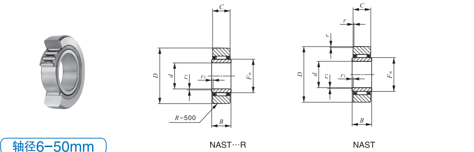
轴径6-50mm
