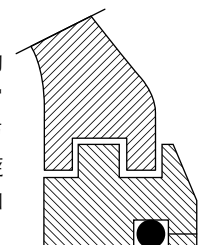
图 28. 迷宫式密封圈
