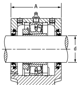
V 形环密封圈
