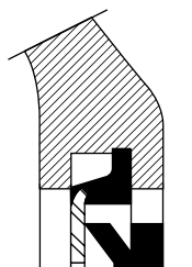
图 27. V 形环密封圈
