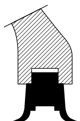
图 26. 双唇式密封圈
