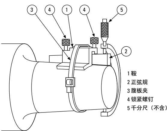
图 50. 正弦规的部件
