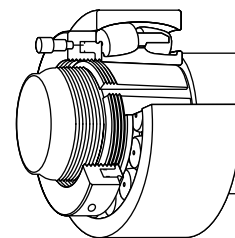
图 54. 用于取下退卸套的液压螺母
