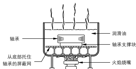
图 16. 热膨胀方法
