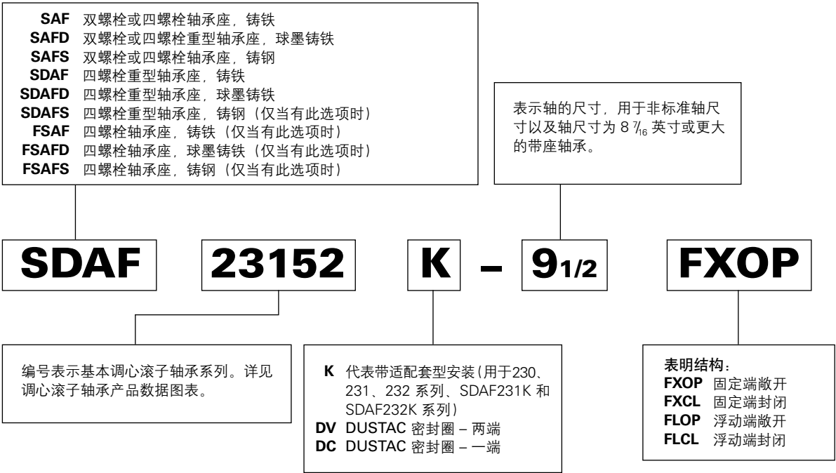
图 47. 轴承座
