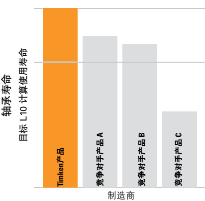
22212EJW33 Timken® SRB与优质竞争对手产品对比。测试条件：负荷 – 50% 额定动载荷；速度 – 2700rpm。
