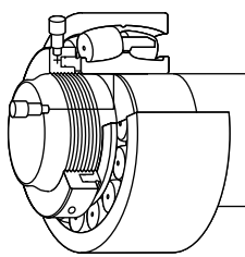
图 52. 用于将轴承安装到锥形轴颈上的液压螺母
