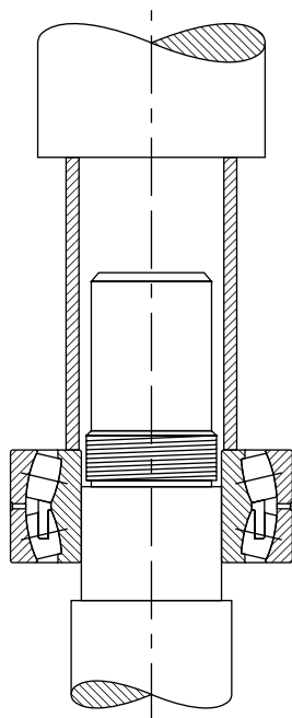
图 17. 手扳冲压法
