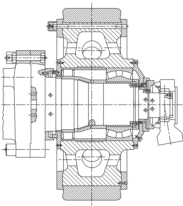
图 10. 磨煤机磨辊
