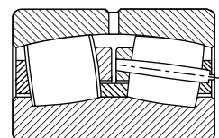
图 8. 销式保持架
