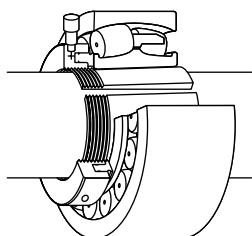
图 51. 用于将轴承安装到紧定套上的液压螺母
