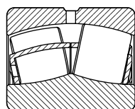
图 2. EJ 轴承
