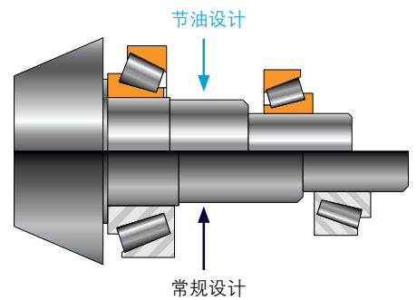
图4. 使用较小的轴承, 可减小系统尺寸。主减轴和基座材料更少, 节省成本和重量
