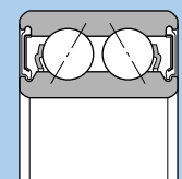
Non-contact sealed type (LLM)
