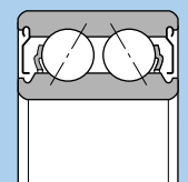
Shielded type (ZZ)
