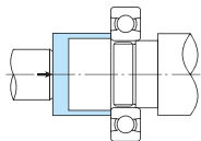
图8.42 内圈的压配合
