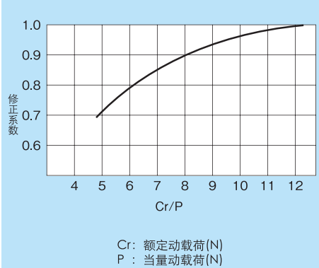
图8.38.1 对轴承载荷的修正系数
