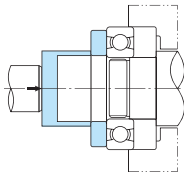
图8.43 内外圈的同时配合
