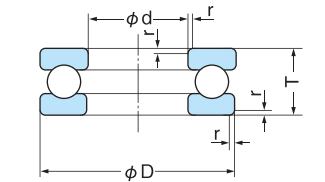
图4.3 单向推力球轴承
