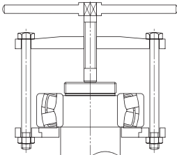
图8.53 专用拉马
