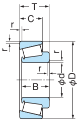
图4.2 圆锥滚子轴承
