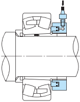
图8.45 液压螺母
