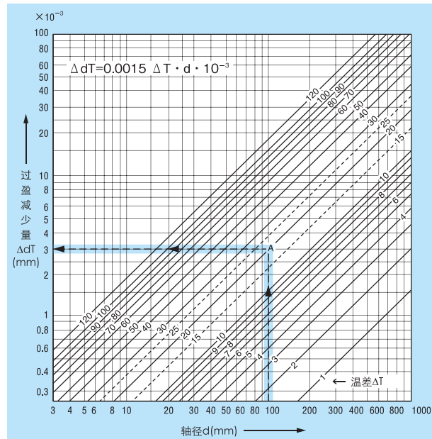
图8.2 由于温差引起内圈过盈的减少
