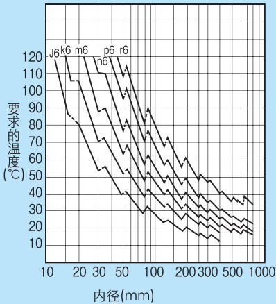
图8.44 要求的膨胀热
