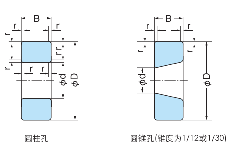
图4.1 相心轴承 (圆锥滚子轴承除外)
