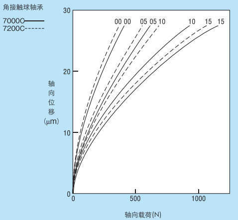
图8.4 向载荷与轴向位移
