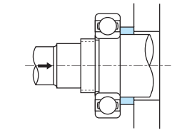
图8.50 使用压机拆卸轴承
