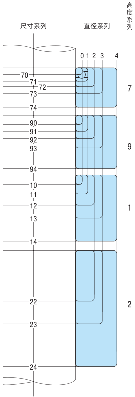
图4.7 推力轴承尺寸系列的图示
