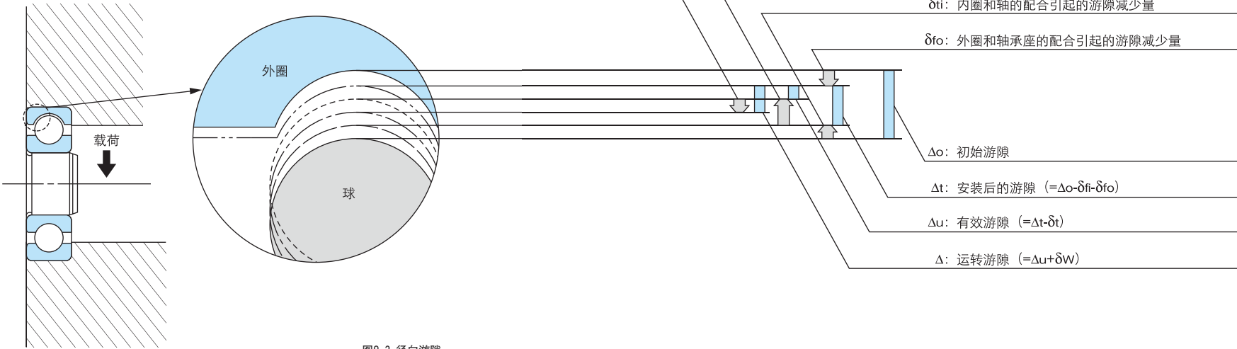
图8.3 径向游隙
