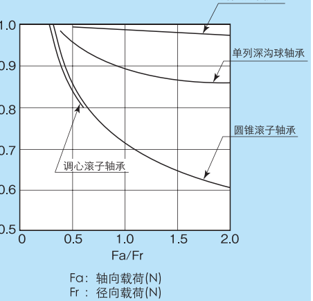
图8.38.2 对Fa/Fr的修正系数
