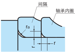
图8.9 使用隔圈时倒角尺寸和圆倒角半径
