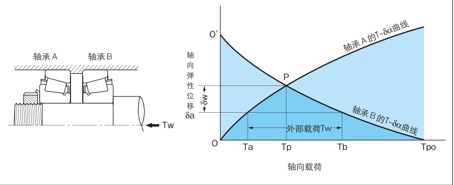
图8.5 定位预载的说明
