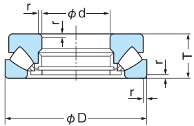
图4.5 推力调心滚子轴承
