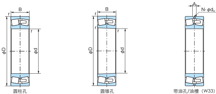
带油孔/油槽 (W33)
