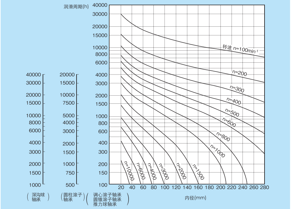
图8.37 润滑脂的润滑周期
