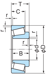
图4.2 圆锥滚子轴承
