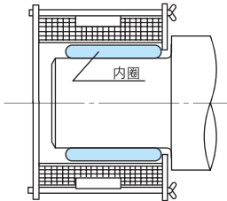
图8.55 用感应加热器拆卸内圈
