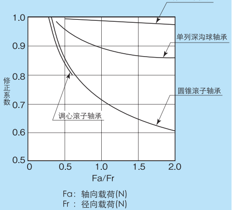
图8.38.2 对Fa/Fr的修正系数
