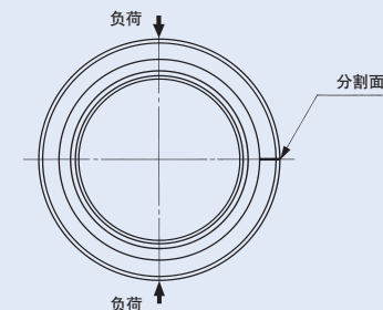
图8 外圈的分割面与负荷方向
