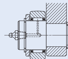
图3 无内圈轴承的安装例
