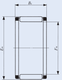
图9 滚针与保持架组件
