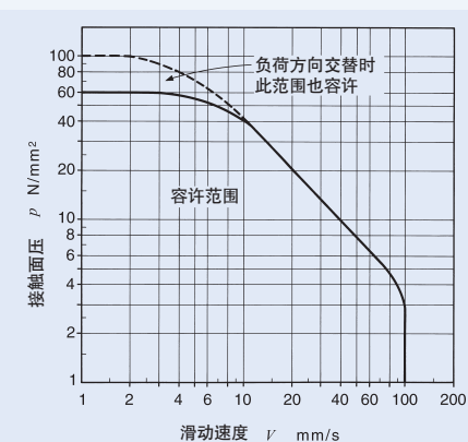
图1 加油式关节轴承的 pV 曲线图
