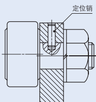
图4 偏心杆端凸轮从动轴承的安装例
