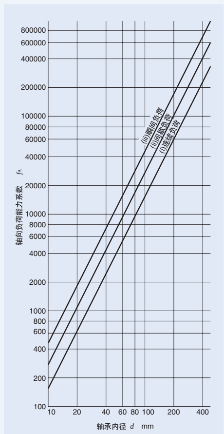
图1 轴向负荷能力系数
