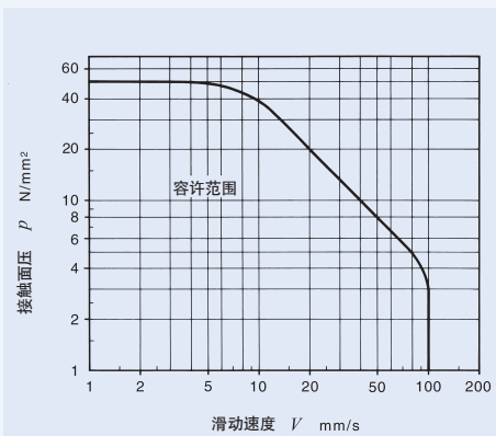
图1 加油式杆端关节轴承的 pV 曲线图
