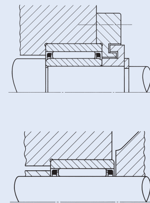
图1 安装例
